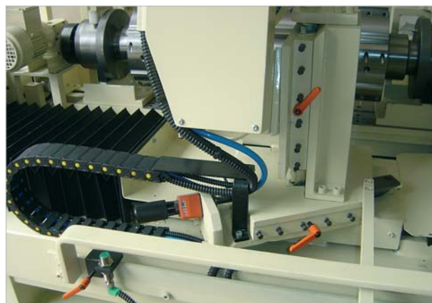
Interruttore di prossimità per limitazione della corsa a seconda della larghezza di lavoro.
