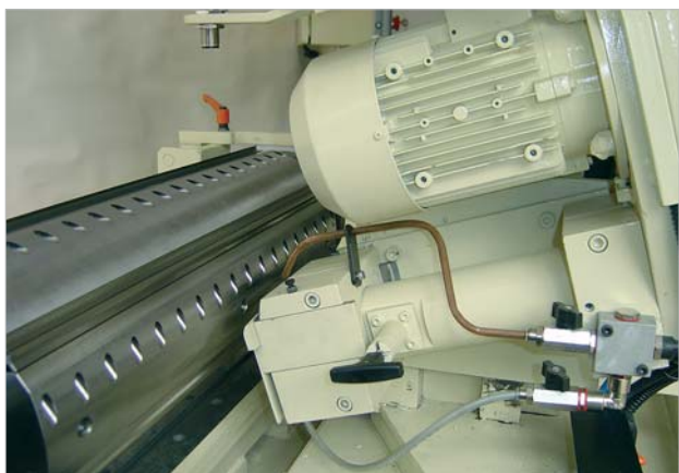
Mola con raffreddamento interno ed esterno per alte prestazioni.
