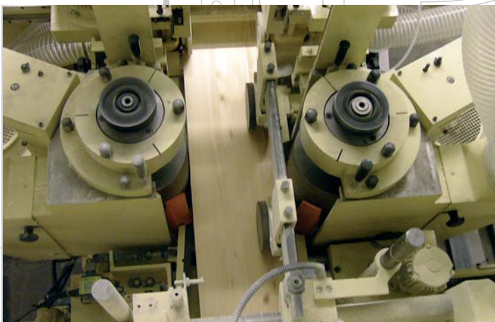
Unità verticali con alberi pialla estraibili (utilizzabili su ambo i lati)
